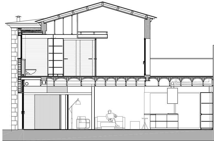
SECCIÓN
