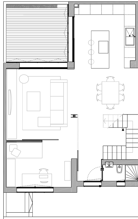
PLANTA BAJA
