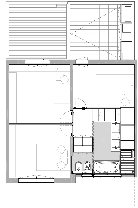
PLANTA PRIMERA
