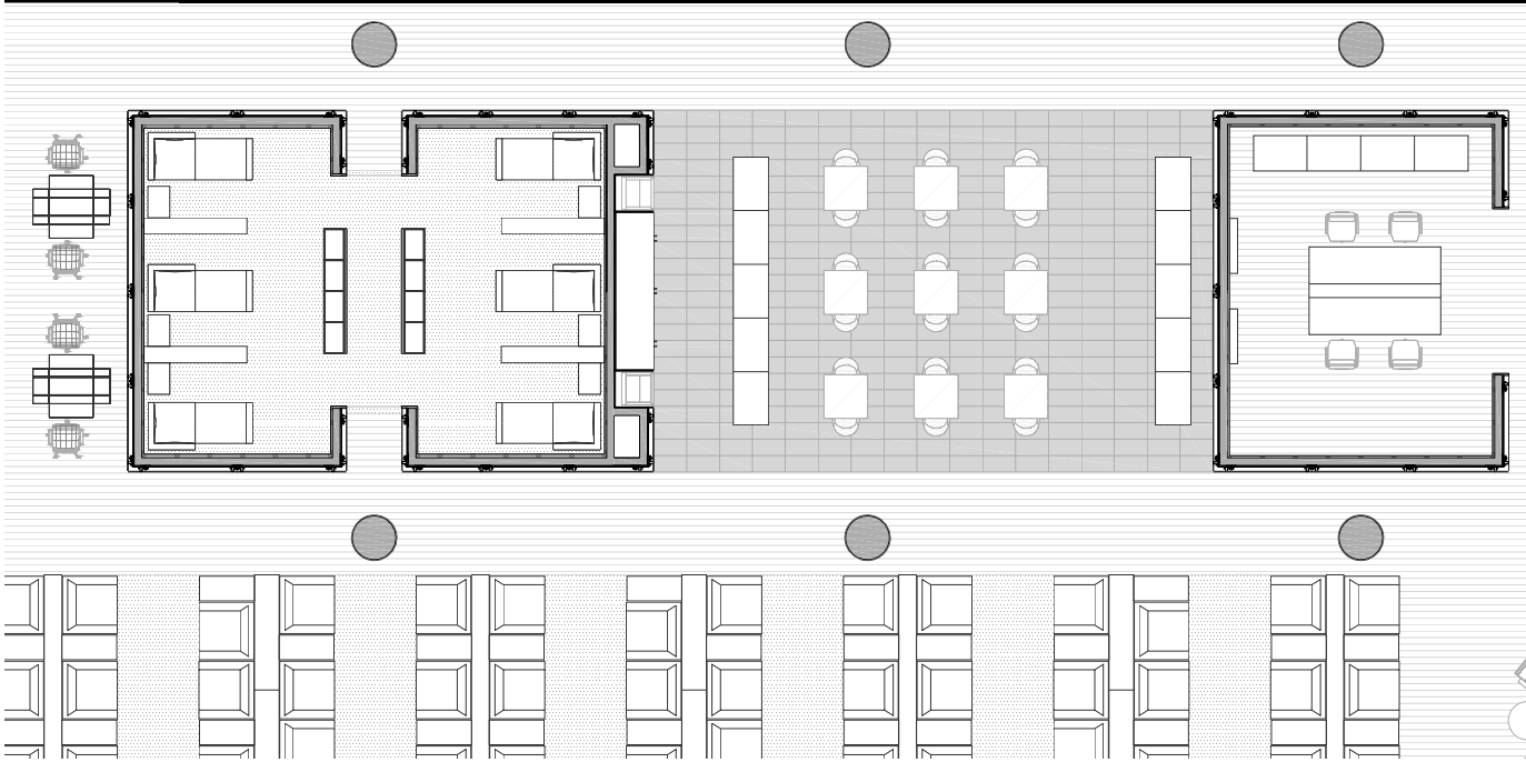
DETALLE DE UNA PARTE DE LA PLANTA
