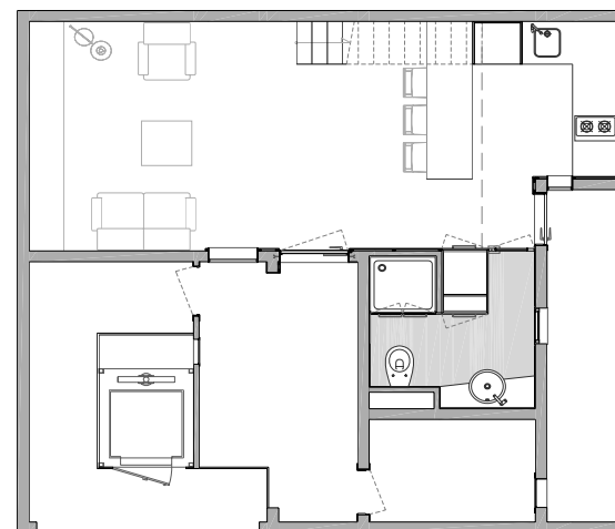
PLANTA BAJA
