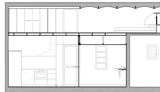
SECCIÓN
